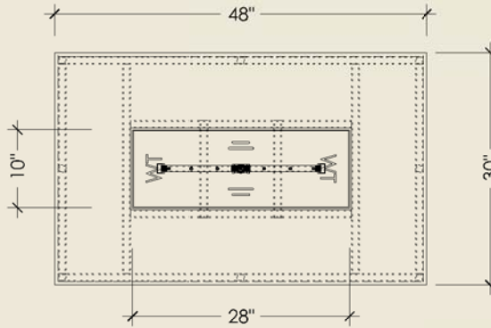
TOP ELEVATION
